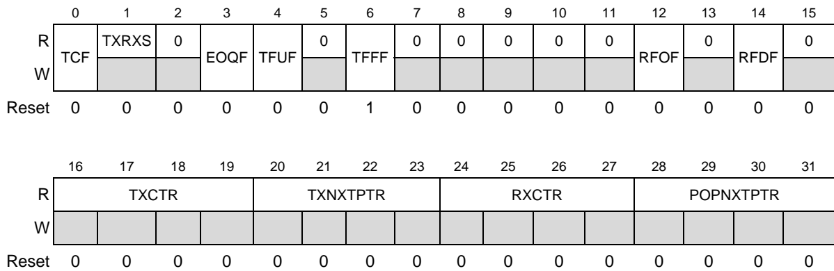
Figure 25-6. DSPI Status Register (DSPI_SR)
