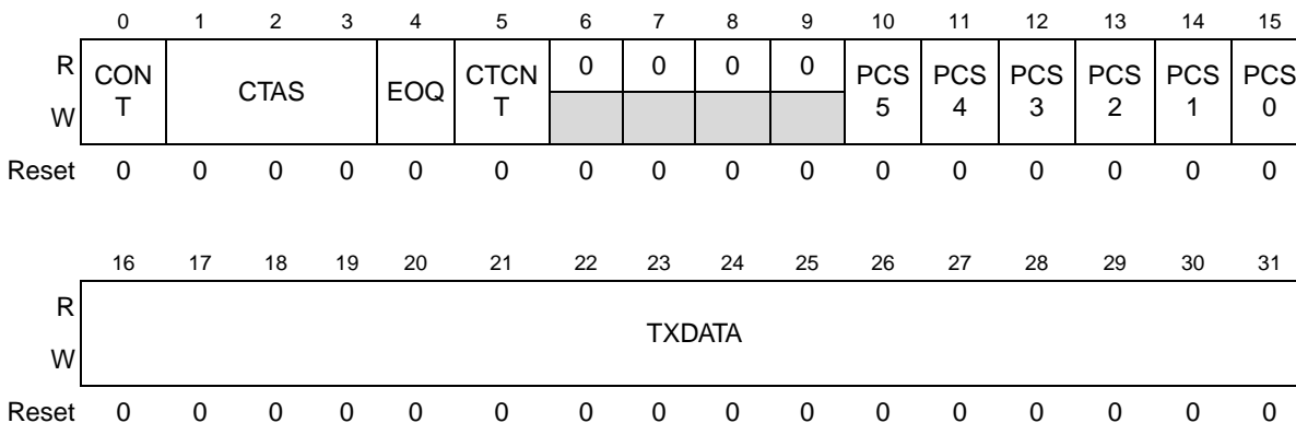
Figure 25-8. DSPI PUSH TX FIFO Register (DSPI_PUSHR)
