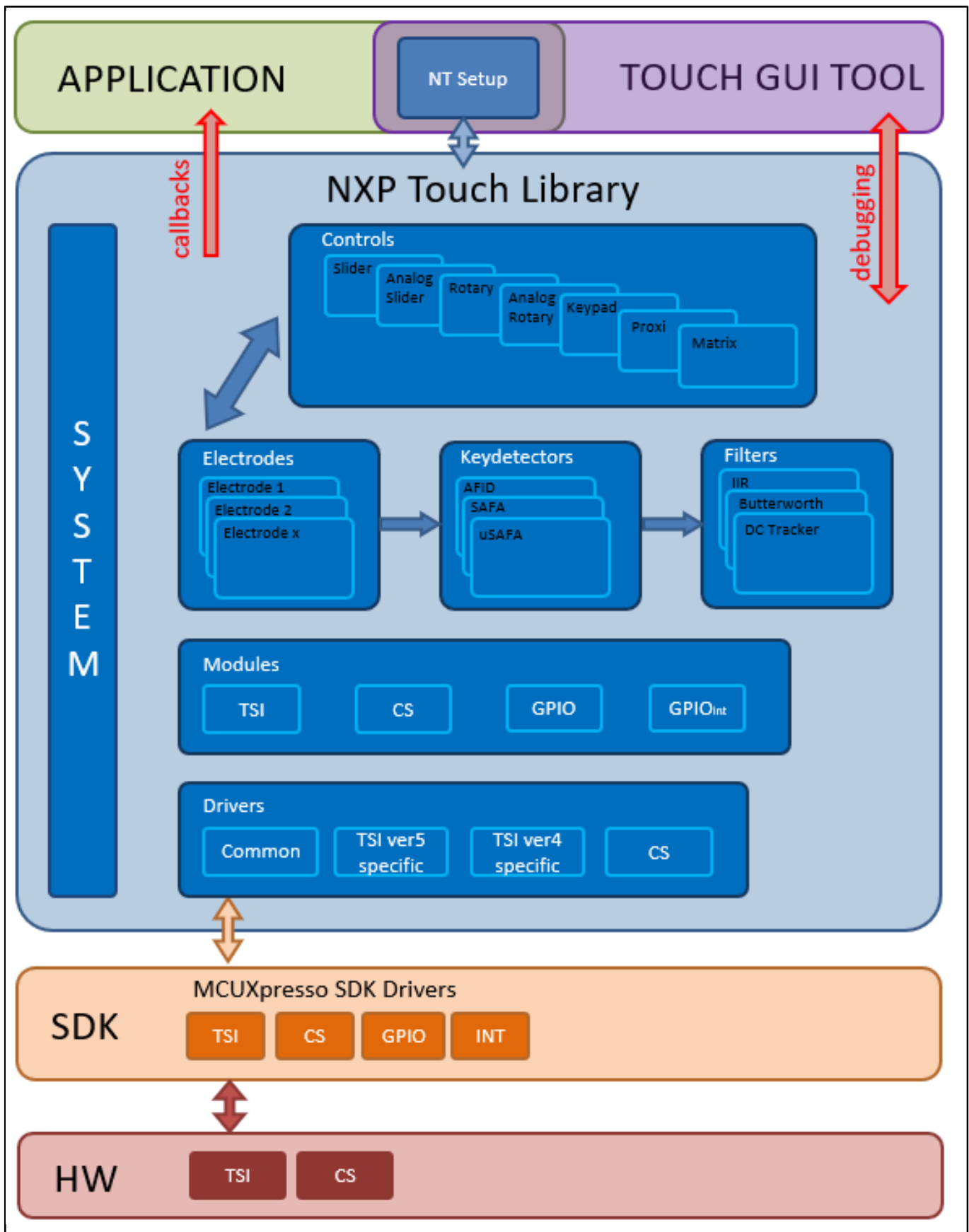
恩智浦®触摸软件结构框图 Block Diagram
